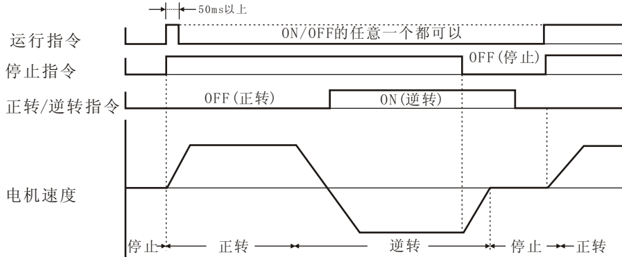
3线制程序的时序图
