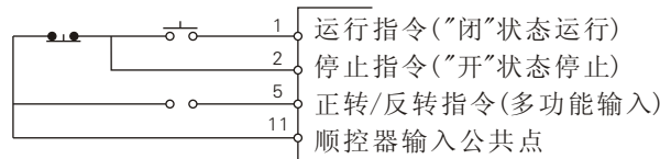
3线制程序的接线举例
