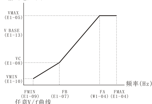
E1-04 (FMAX) > E1-06 (FA) > E1-07 (FB) = E1-09 (FMIN) 输出电压(V)
