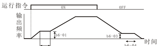
DWELL功能的时序图
